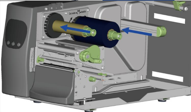
外捲式碳帶安裝方式 (即油墨面朝外)
