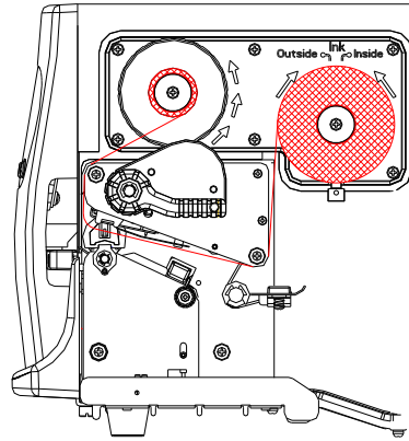
內捲式碳帶安裝方式 (即油墨面朝內)
