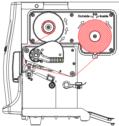
外捲式碳帶安裝方式 (即油墨面朝外)
